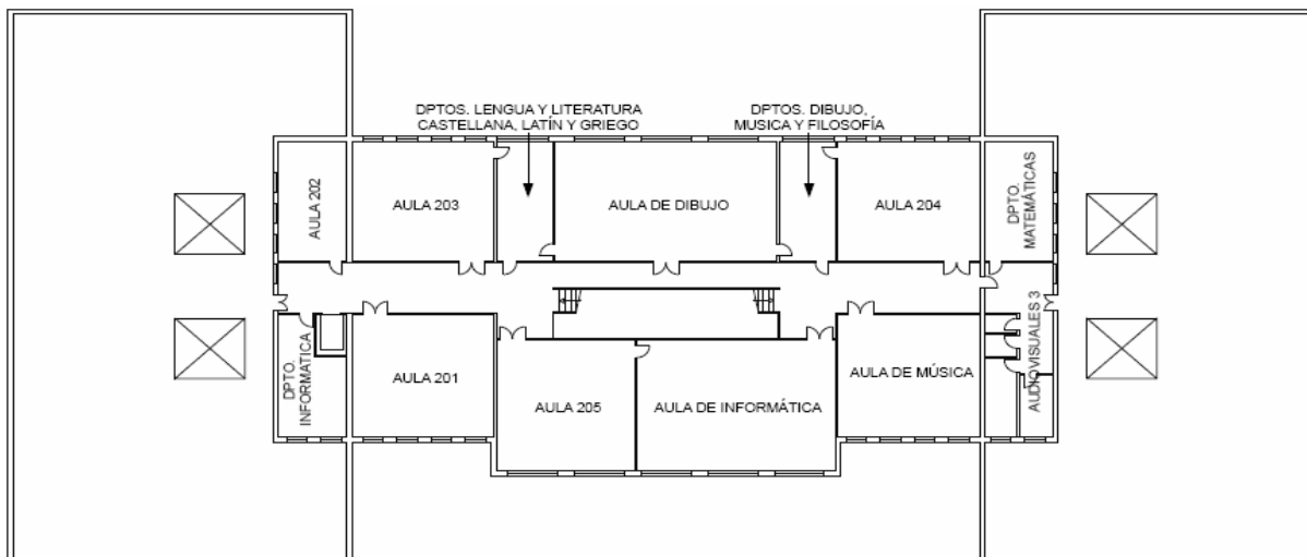
Plano planta segunda:
